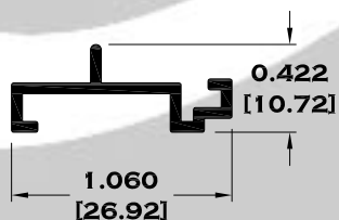
9966 ADAPTADOR MOSQUITERO
