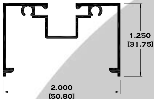
9083 BOLSA
