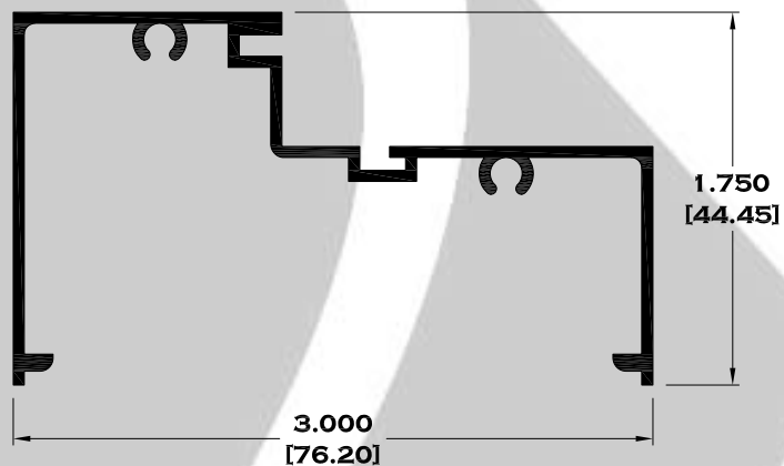
9136 ESCALONADO
