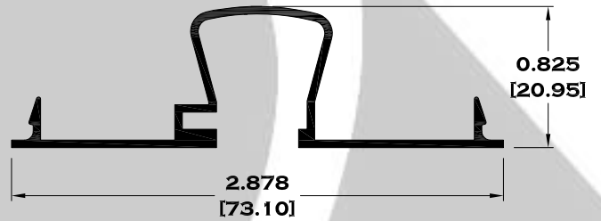
7315 TAPA BOLSA
