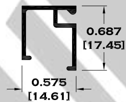
6370 JUNQUILLO
