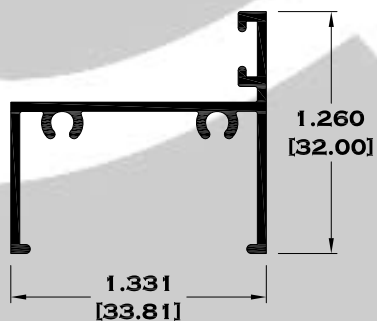
8560 BATIENTE LARGO
