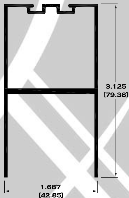
9187 ZOCLO
