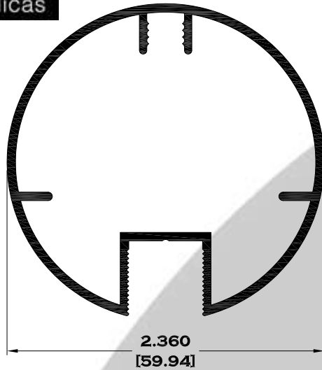
23896 PASAMANOS REDONDO 2"
