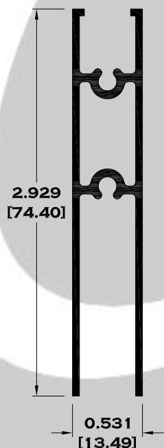
7825 ZOCLO PUERTA
