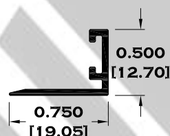
11032 BATIENTE
