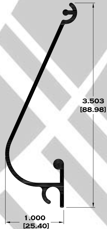
10466 JALADERA
