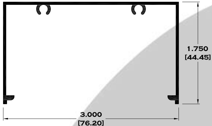
9114 BOLSA LISA
