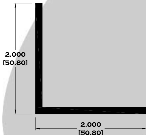
8 ANGULO DE 2" X 2" X 1/8"
