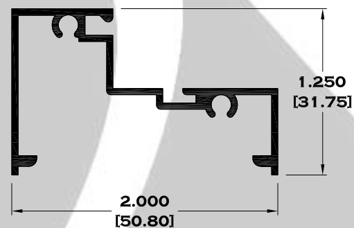
9084 ESCALONADO
