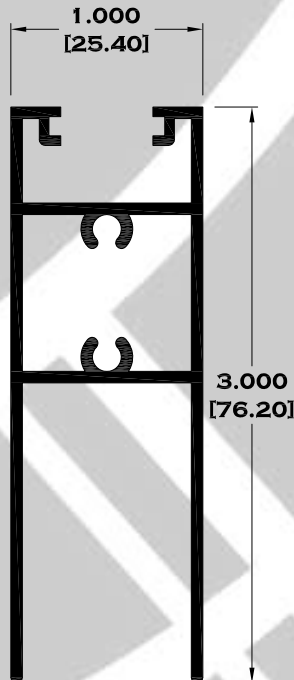
7842 ZOCLO PUERTA
