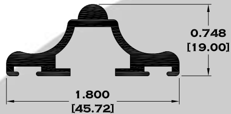
033 MOLDURA
