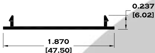
4051 TAPA LISA
