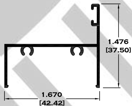
8570 BATIENTE
