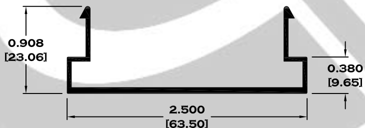
5472 TAPA INTERIOR BÁSICO
