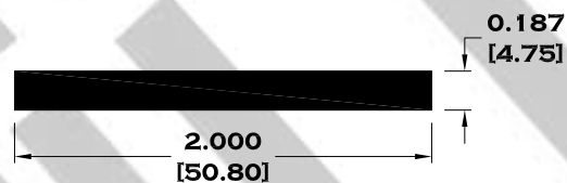
1216 SOLERA DE 2" X \frac{3}{16} "
